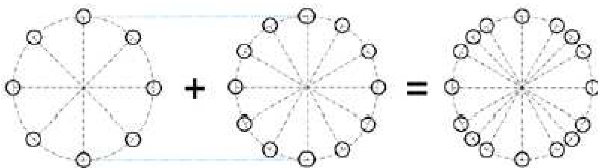
Rozteč šroubů PN 10 8 děr
